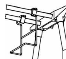
УСТАНОВКА L-ОБРАЗНОГО КРОНШТЕЙНА ДЛЯ СИСТ. БЛОКА НА V-ОБРАЗНЫХ КОННЕКТОРАХ L-TYPE HOLDER FOR CPU WITH V-CONNECTORS INSTALLATION
